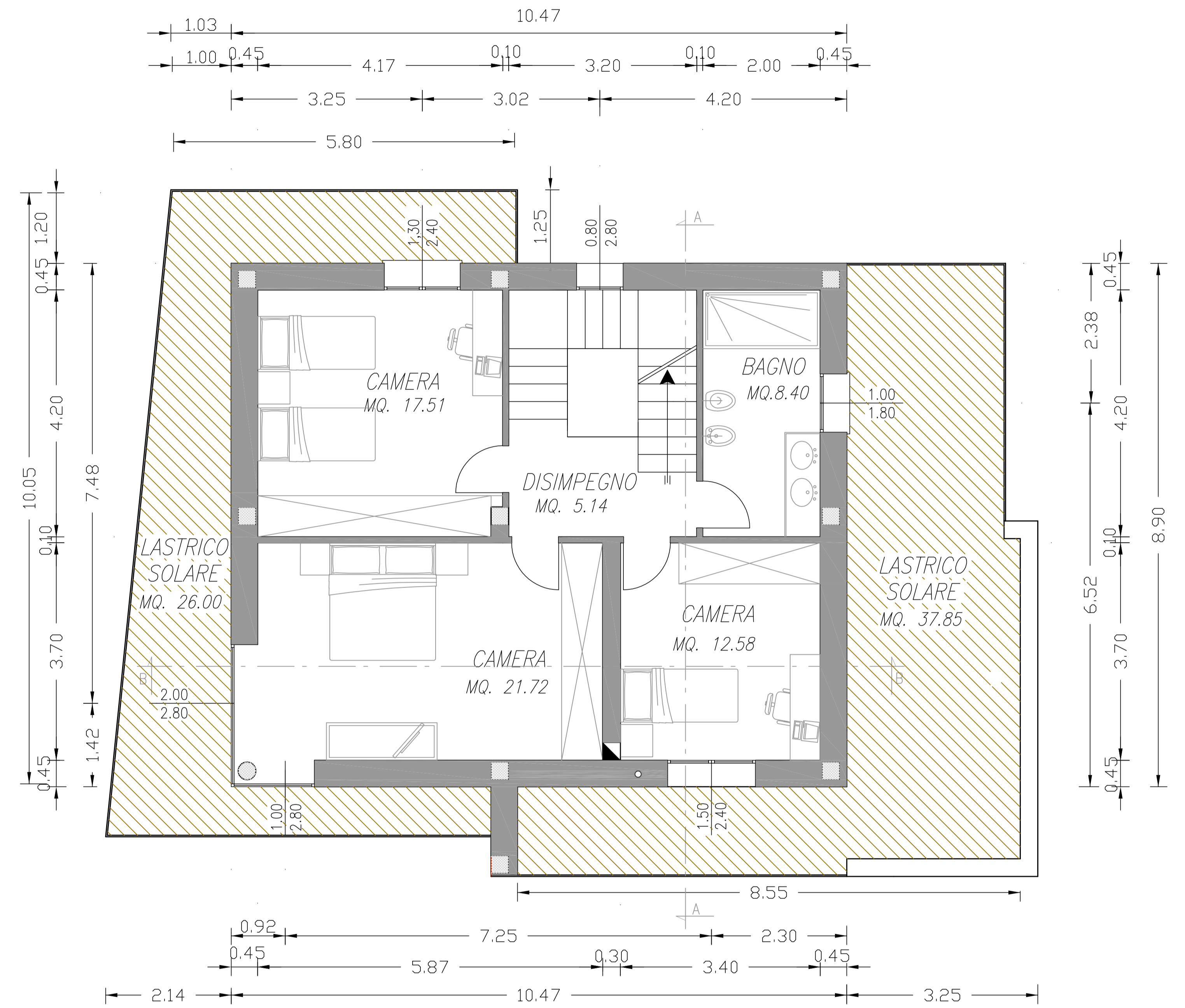
PIANO PRIMO H=2.80
